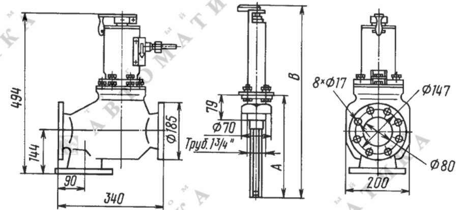
Габаритные размеры терморегулятора РТЦД-80-Р
