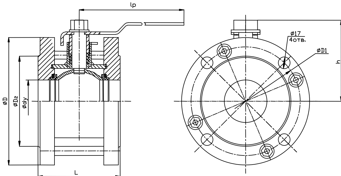
Рисунок 1. Общий вид крана
