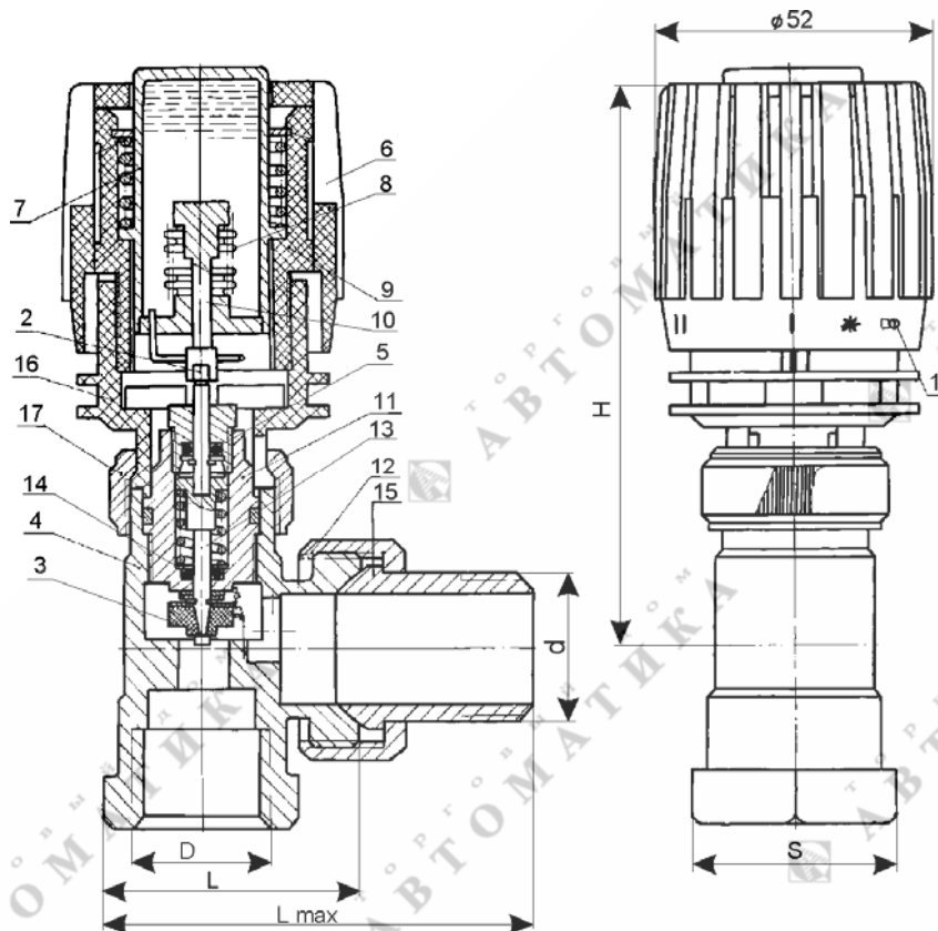
Рис. 2 (СНИЦ. 423.117.019-02; 03)
