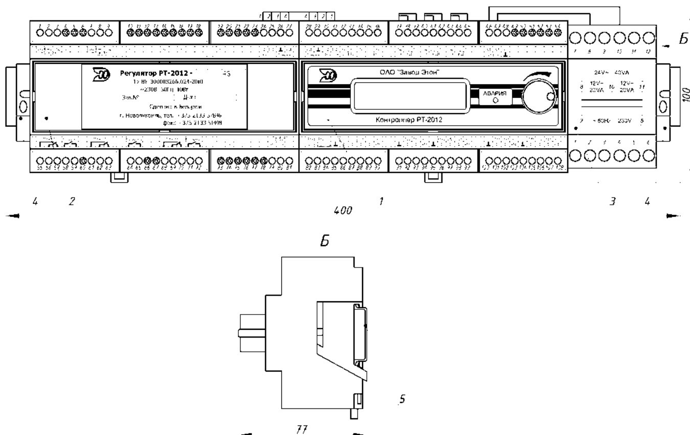
Рисунок 1 - Внешний вид контроллера
