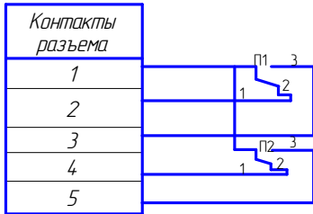
Схема принципиальная электрическая
