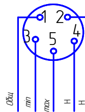
Схема внешних соединений
