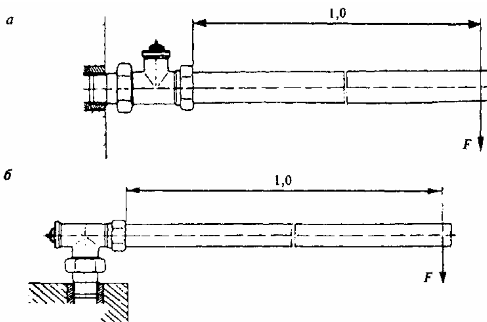
a - проходной клапан; b - угловой клапан
