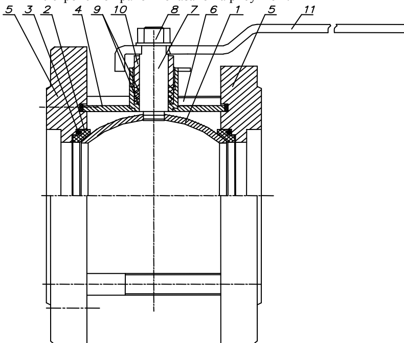
Рисунок 1. Общее устройство крана
