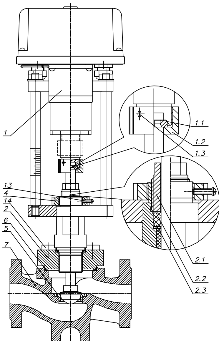
Рисунок 1 Общее устройство клапана КЗР 25/XX.Б-XX
